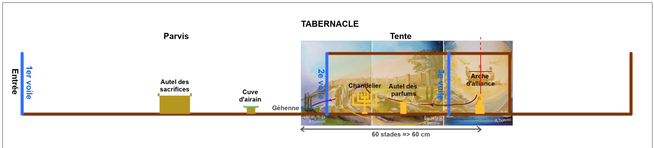
Juxtaposition du triptyque et du Tabernacle (vue de profil)
